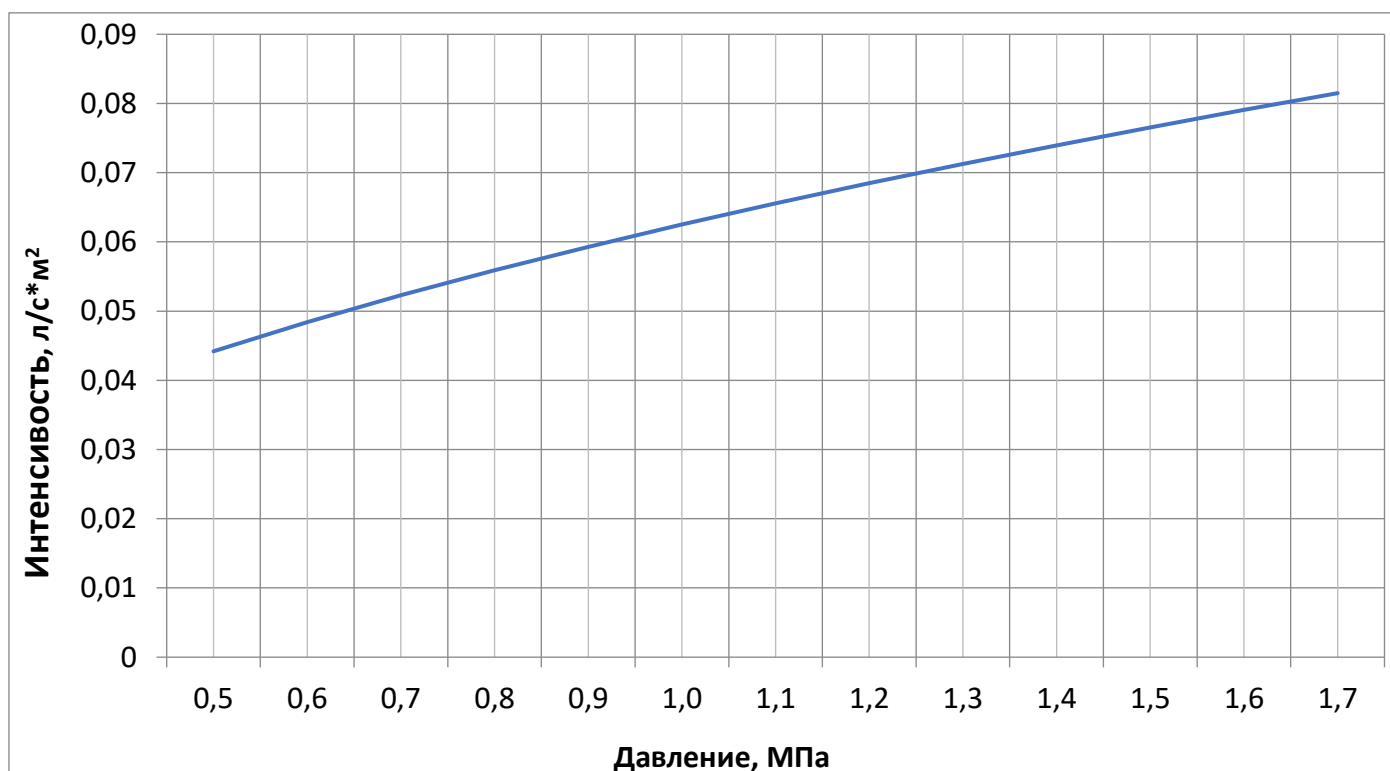
График зависимости интенсивности орошения от давления на площади 16 м 2 , защищаемой одним оросителем с высоты 2,5 м
